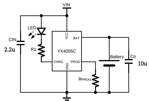
图 1. 典型应用电路
