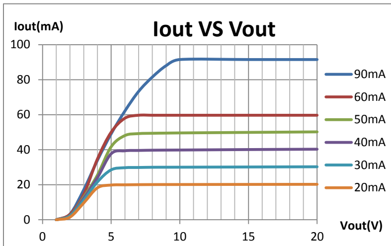
图 1. SM2082EG 恒流曲线图
