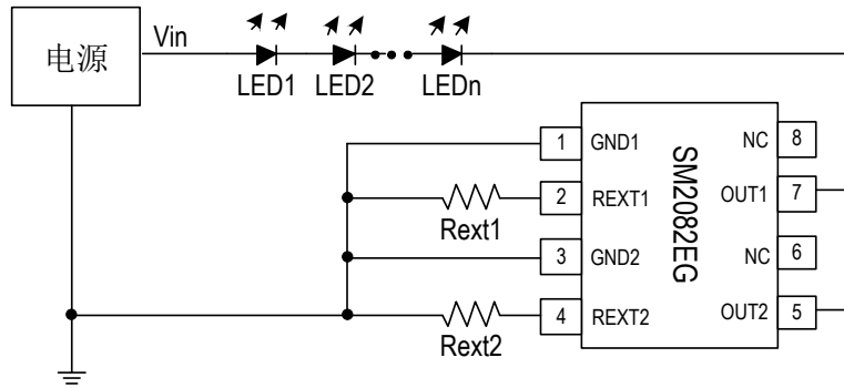
图 3. SM2082EG 应用电路原理图
